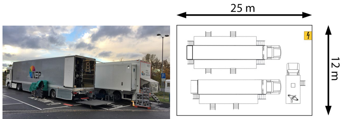
Abbildung 14: TV-Compound / Maße
