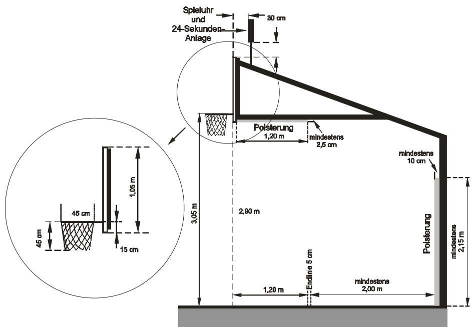
Abbildung 3: Standkorbanlage
