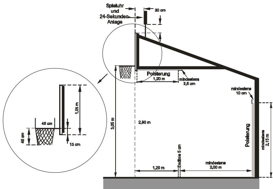
Abbildung 3: Standkorbanlage
